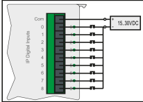
Girişlere kuru kontak bağlanılması npn
