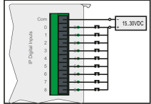
Girişlere kuru kontak bağlanılması. npn
